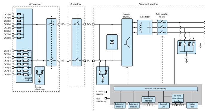
Блок-диаграмма PRO-33.0-TL-OUTD
